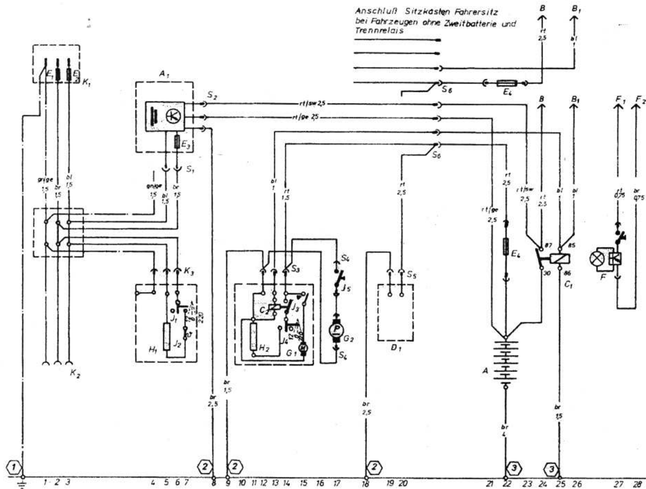
Schaltplan 12V/220V
